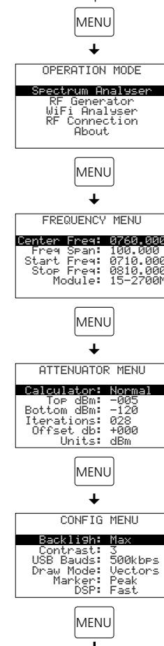
Fig. 4 Struttura del menù
