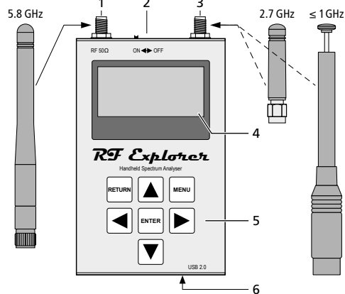
Schéma 1 Branchements et éléments
