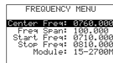
Fig. 6 Menù frequenze
