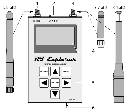
Abb. 1 Anschlüsse und Bedienelemente
