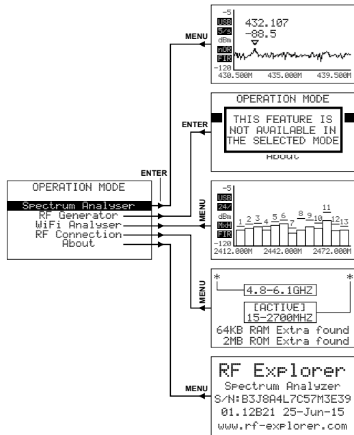
Schéma 5 Operation Mode (Menu mode fonctionnement)
