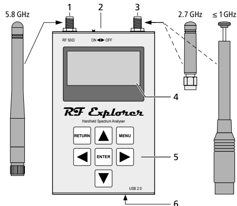
Fig. 1 Collegamento e elementi di comando
